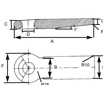
Type Belge Belgium type Belgischer Typ Belgisch type Tipo Belga
