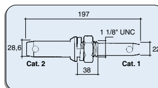
68/8127-212 (1167-2) Avec écrou et rondelle Complete with nut and washer
