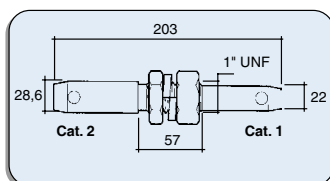
68/8127-211 (1165-1) Avec écrou et rondelle Complete with nut and washer
